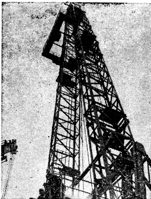
宝鸡石油机械厂研究所设计研制的抽油机、螺旋量规获国家银质奖，吊环荣获国家金质奖。并为我国海洋钻井船研制了动态井架，为发展我国石油工业做出了贡献。图为架井局部。(宝鸡市国庆摄影展览办公室供稿)
