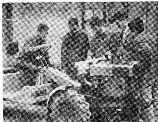
陕西拖拉机厂科技人员，最近将原为二型手扶拖拉机的把手式转向机构革新为方向盘式，操纵比以前灵活、安全，很受司机欢迎。 无知 摄
