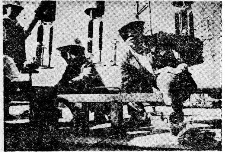
西北电建一公司福州火电厂工地电气高压班副班长魏运汉，在安装开压站设备时发明了基础找平架，解决了找水平难的问题，为设备安装赢得了时间。日方技术人员对此曾大加赞赏。这是魏师傅（右一）正在用基础找平架工作。 柳影摄
