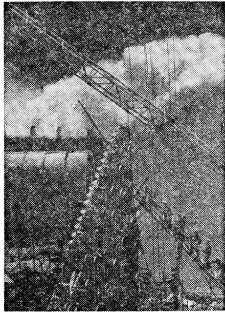
堪称万里黄河第一坝的龙羊峡水电站位于青海省龙羊峡谷进口约两公里处，设计坝高178米，共装机4台，单机容量为32万千瓦，库容为247亿立方米。
