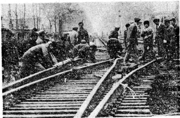
为提高列车的通过能力,由郑州铁路局西安工程公司承担施工任务的西安至宝鸡区段铁路电气化改造工程已在沿线各车站全面展开。图为西安工程一段工人在绛帐车站增铺岔线。侯登科摄
