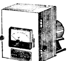
LTD-1 型勵磁式勵磁調節器
