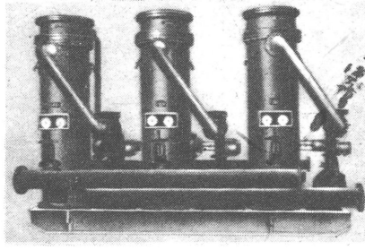
图为YSS型油水冷却器
