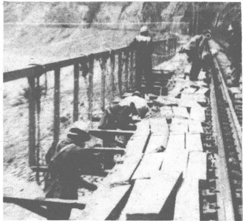
8月份,宝天山区连降大雨,拓石工务段的职工发扬工人阶级战天斗地的大无畏精神,对沿线的关键处所和重点设备进行重点整治,确保了行车安全。图为伯阳桥隧工区在维修加固钢梁支架。
