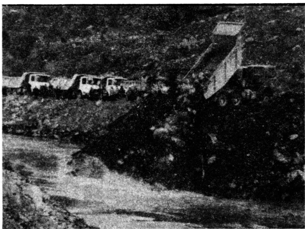
11月29日10时45分，国家重点工程宝珠寺水电站截流成功。该电站位于川、陕交界的广元市境内，总库容25.5亿立方，装机容量70万千瓦时。陈玉恒 李卫华摄
