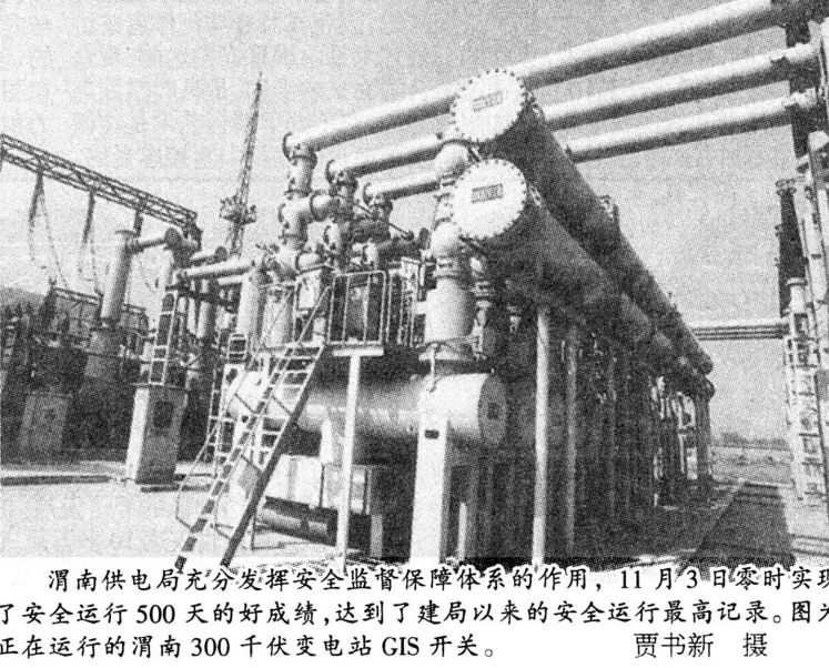
渭南供电局充分发挥安全监管保障体系的作用,11月3日零时实现了安全运行500天的好成绩,达到了建局以来的安全运行最高记录。图为正在运行的渭南300千伏变电站GIS开关。
