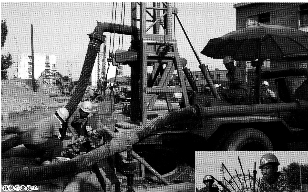
钻机作业施工
